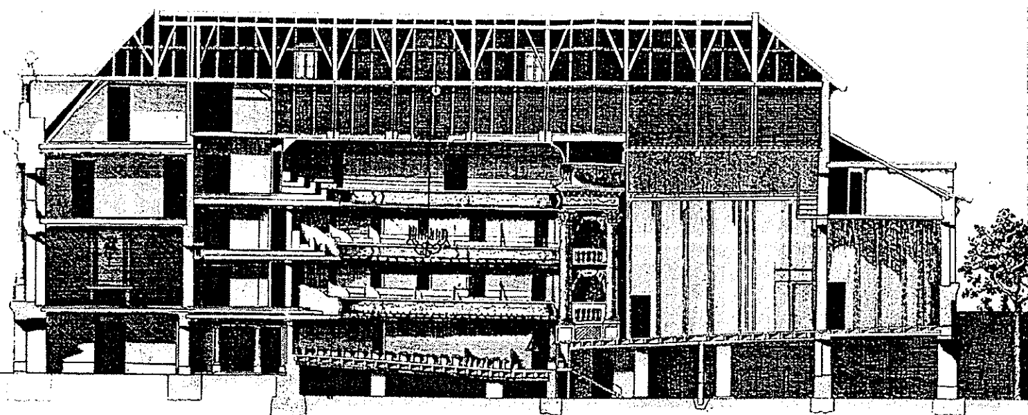
Coupe et profil pris sur la ligne AB des Plans de la Salle de Spectacle, exécutée à Genève, en 1783.
