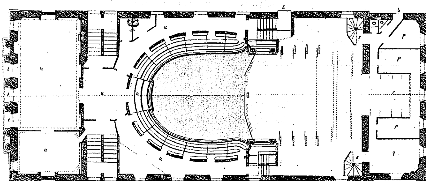
Plan du premier étage.
