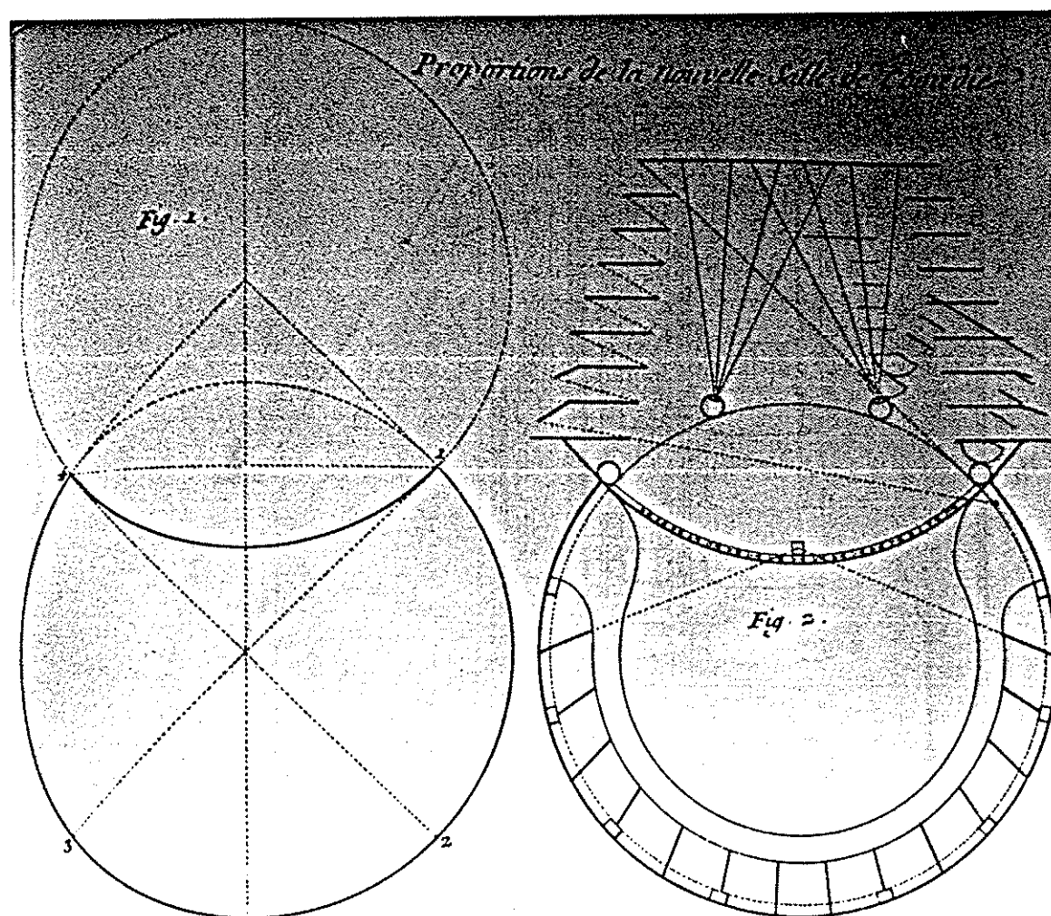
Proportions des trois Théâtres modernes réduits sur la même Echelle.
